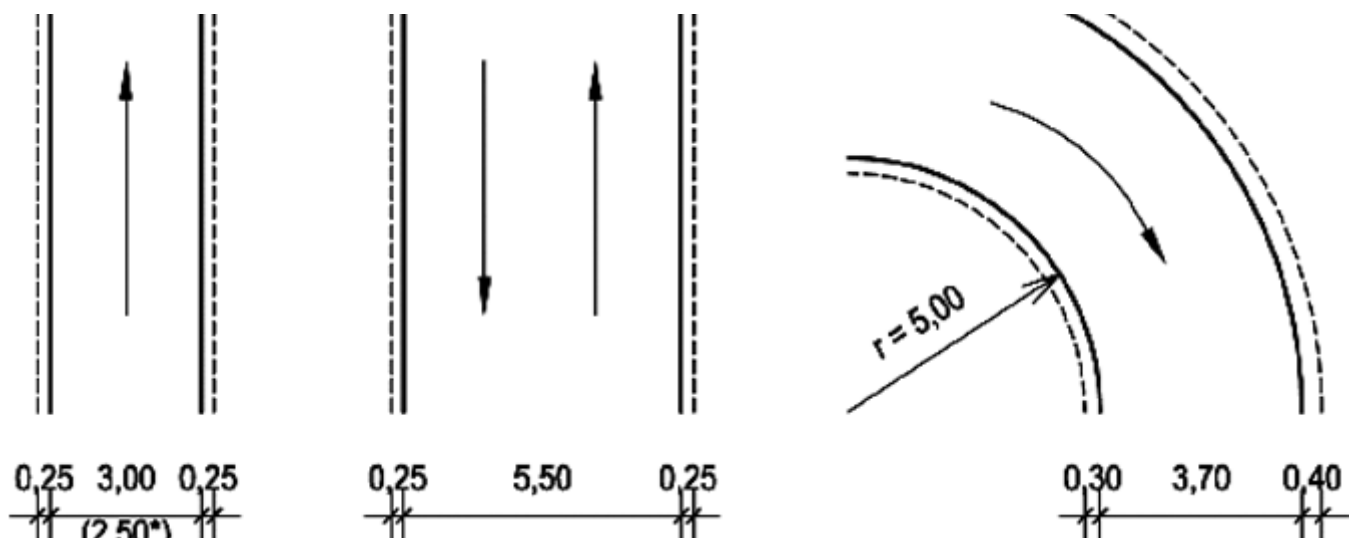
1. ábra: az álláshelyekhez vezető közlekedési út egyenes és íves szakaszai (rendszeres gyalogosforgalom nélkül)
